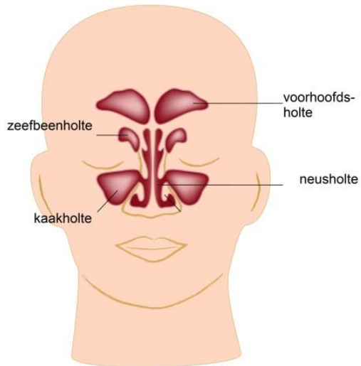
Afbeelding 1: de zeefbeenhollen
